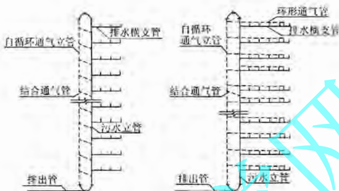
图2 自循环通气形式
