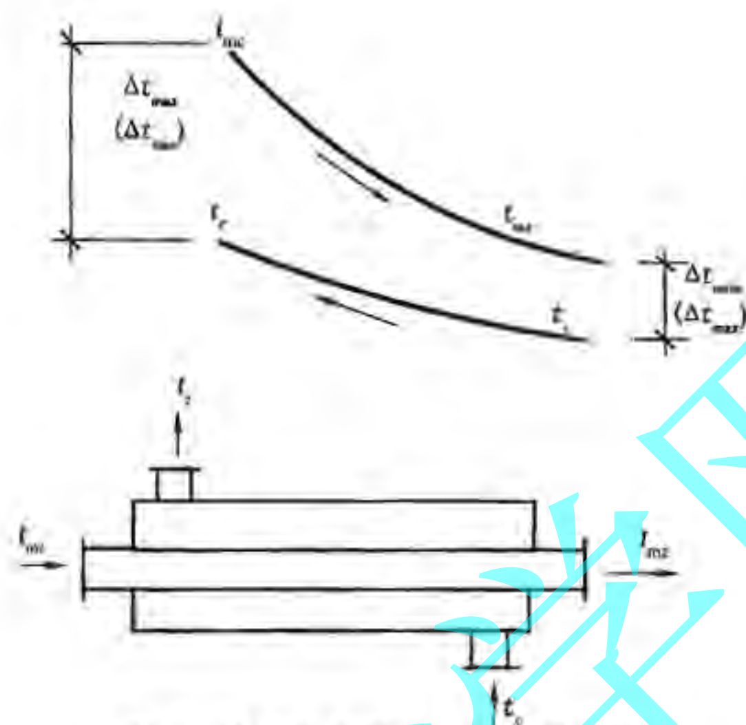
图4 快速换热器水加热工况示意
