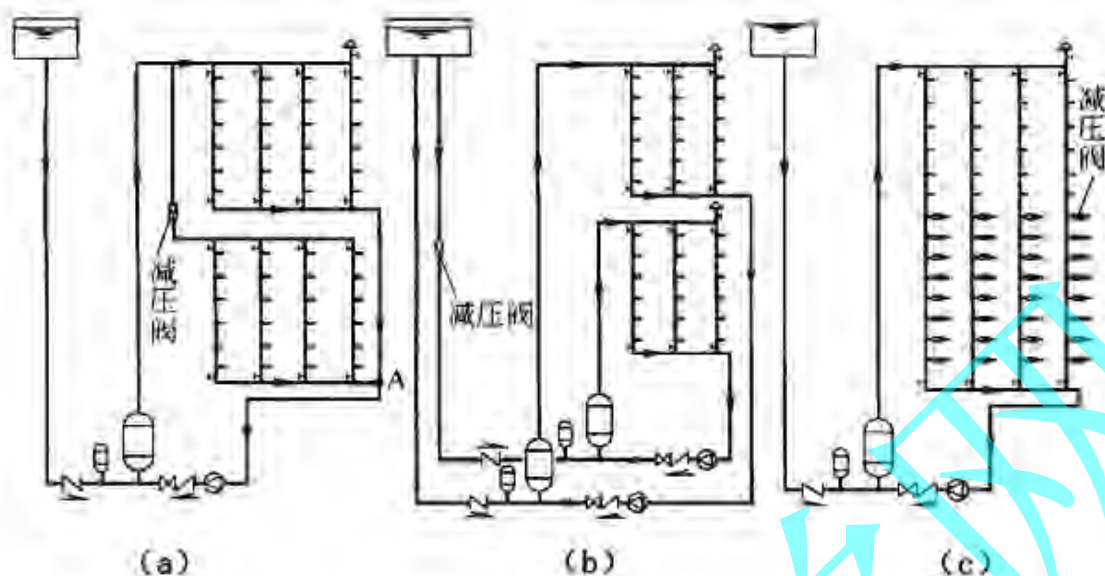
图3 减压阀设置
